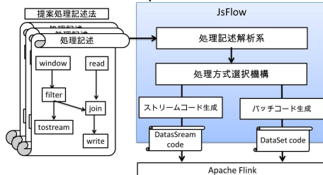
図 4: JsFlow 全体図
