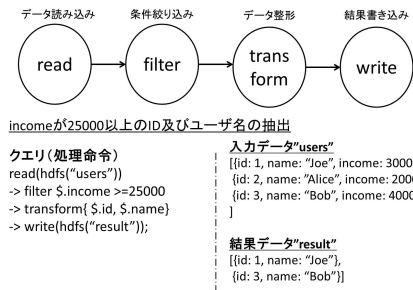
図 3: Jaql 処理記述例
