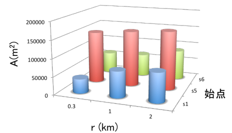
図 12: 始点と r を固定した場合の A の平均値
