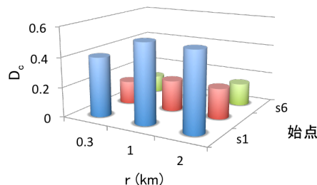
図 19: d_{min} に対する D_c の値
