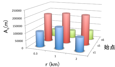
図 17: d_{max} に対する A_c の値
