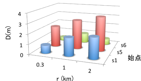
図 21: 始点と r を固定した場合の D_c の平均値
