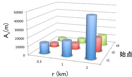
図 16: d_{min} に対する A_c の値
