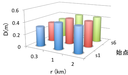
図 13: d_{min} に対する D の値
