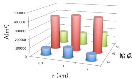
図 11: d_{max} に対する A の値
