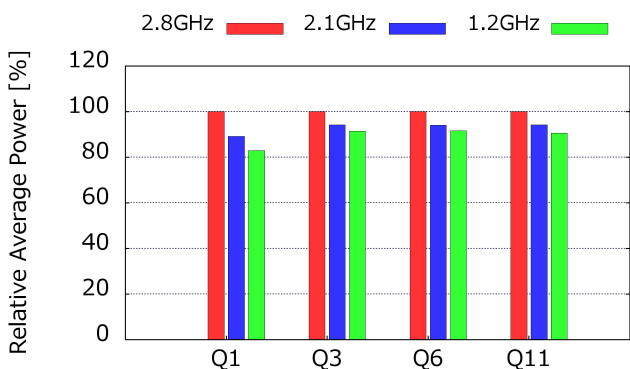
図 11: TPC-H の各問合せの多重度 4 による同時実行時の消費電力 (2.8GHz の時基準)
