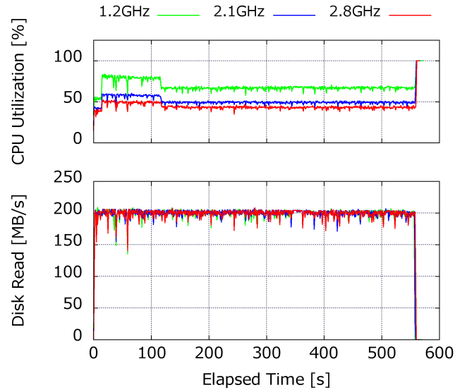
図 6: Q3 を単独実行時の CPU 使用率とディスク速度の経時変化
