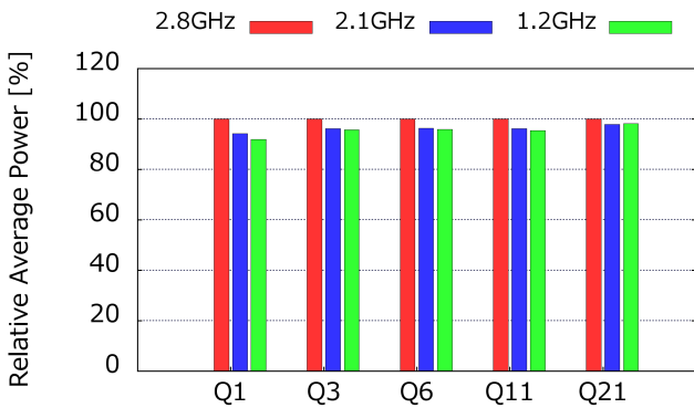
図 3: TPC-H の各問合せの単独実行時の消費電力 (2.8GHz の時からの相対値)
