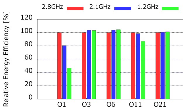
図 1: TPC-H の各問合せの単独実行時のエネルギー効率 (2.8GHz の時からの相対値)
