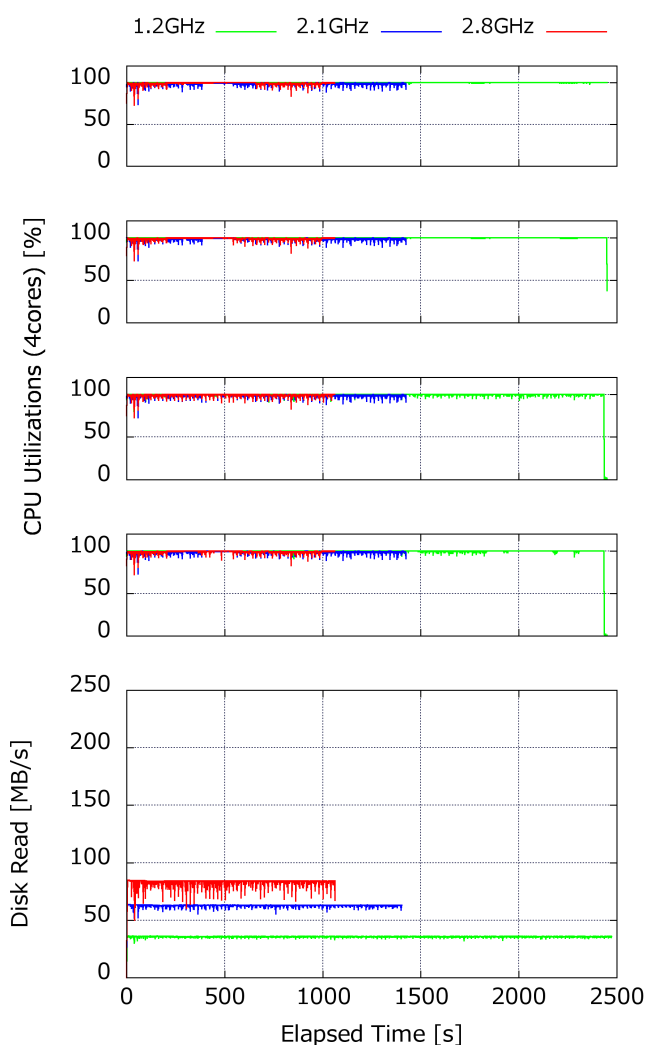
図 12: Q1 を多重度 4 で同時実行時の CPU 使用率とディスク速度の経時変化
