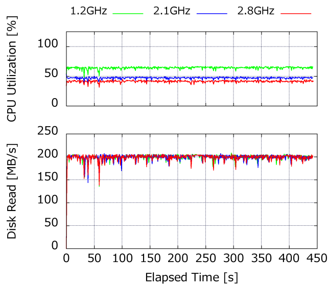
図 7: Q6 を単独実行時の CPU 使用率とディスク速度の経時変化
