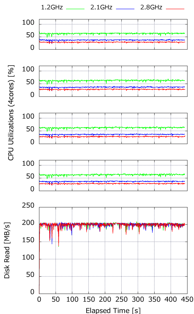
図 13: Q6 を多重度 4 で同時実行時の CPU 使用率とディスク速度の経時変化
