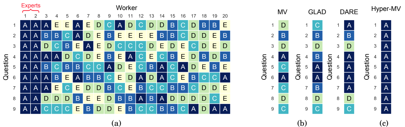
図 2: 従来法が失敗する例: (a) ‘A’~‘E’の5つの選択肢を持つ9件の多肢選択式問題（全て正解は‘A’）に対し、20名のワーカーから回答を集める。20名中2名は専門家であり、全ての問題に正答する。残りのワーカーは、5つの選択肢からランダムに一つ選んで回答する。(b) 多数決では正解は得られず、より高度な統計的手法（GLAD [18], DARE [1]）でも多くの場合に失敗する。(c) 提案法（HYPER-MV）では、全ての問題で正解を得ることができる。
