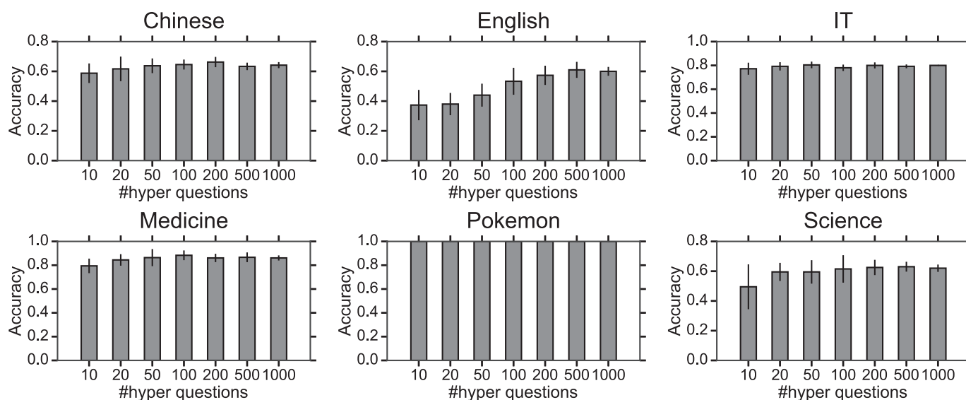
図 6: 超問題の数が HYPER-MV ( k = 5 ) の正答率に与える影響。10 種類の超問題集合に手法を適用した場合の、正答率の平均と標準偏差を示している。超問題の数が 200 以上の場合、すべてのデータセットで正答率が安定している。
