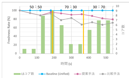
図 14 実験 2 : OLTP 処理性能
