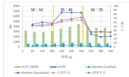
図 12 実験 2：OLTP 処理性能
