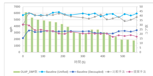
図10 実験 1 : OLAP 処理性能
