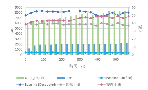
図9 実験 1 : OLTP 処理性能
