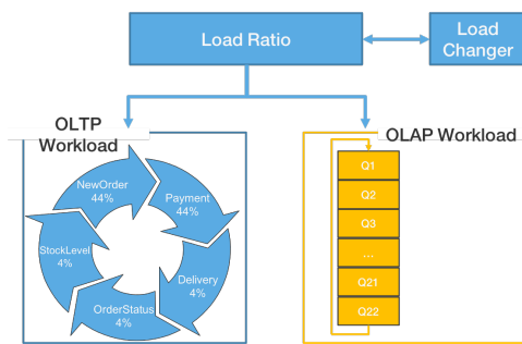
図8 CH-benCHmark+ 概要図
