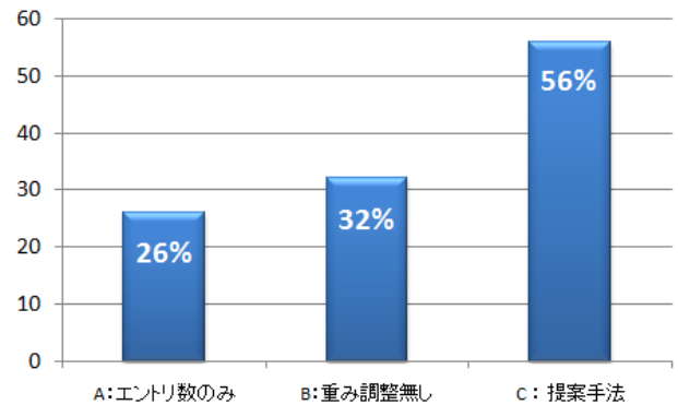
図5 各種マニアランキングによるランキング上位10件に対する適合率
