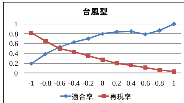
図 12 適合率と再現率の推移(台風型)
