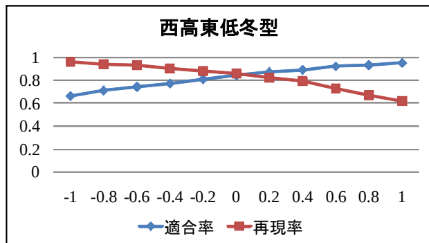
図 7 適合率と再現率の推移(西高東低冬型)
