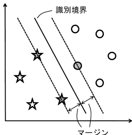
図2 SVMによる線形分離
