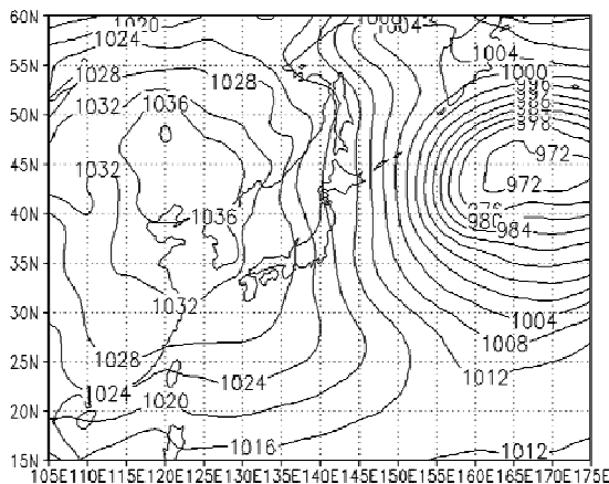
図1 対象領域の海面更正気圧
