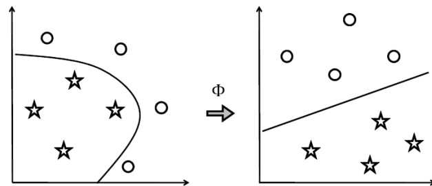
図3 非線形分離
